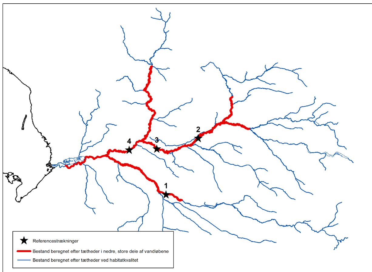
Figur 2.1. Figuren viser hvor i vandsystemet laksebestandsstørrelsen blev beregnet ved anvendelse af habitatkvaliteten (GLHS) – blå streg, og hvor de blev beregnet ud fra tætheder på typiske referencestrækninger i de større dele af vandløbssystemet - rød streg. Placeringen af referencestrækningerne 1-4 er markeret med stjerne. Tallene henviser til de enkelte referencestrækninger, se beskrivelser af disse og opgørelsesmetode i teksten.
