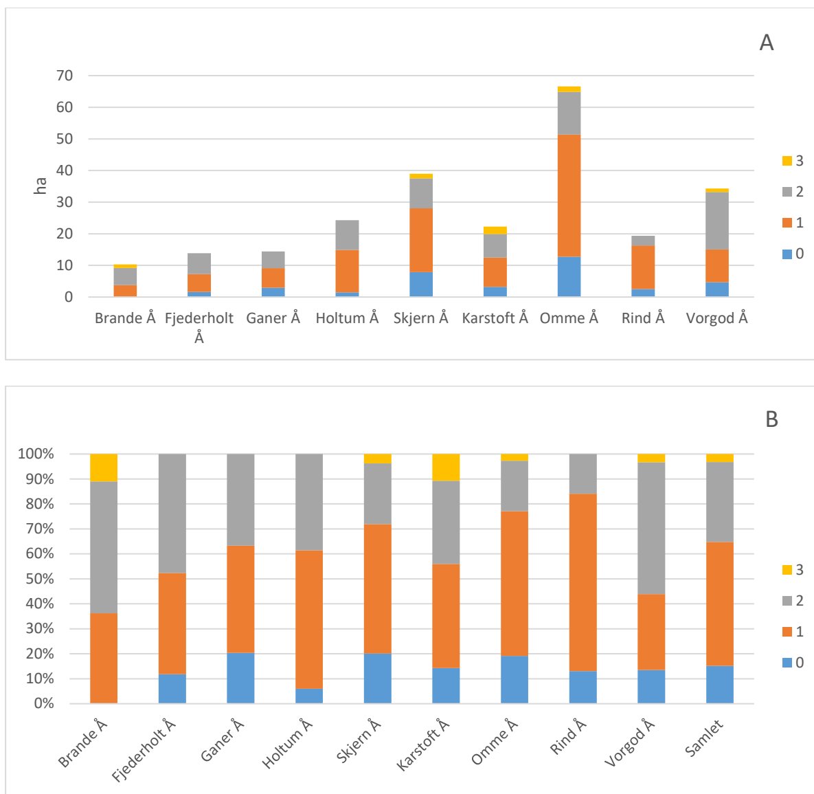
Figur 3.2. A. Arealer (Ha) med forekomst af forskellige habitatkvaliteter (GLHS) for ½-års laks i vandløbene i Skjern Å-systemet. B. Relativ arealmæssig fordeling af habitatkvalitet (GLHS) i vandløbene i Skjern Å-systemet.
